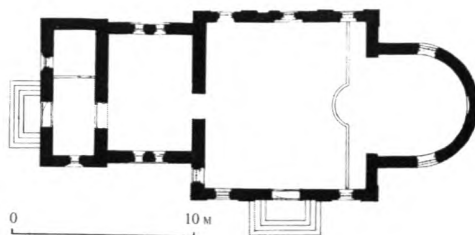
План в уровне входов
