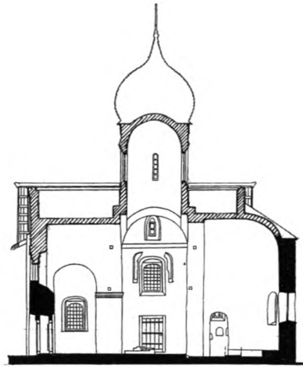
Продольный разрез. Вид на север
