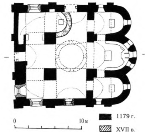
План в уровне входов
